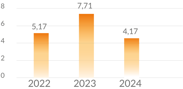
Gráfica 34. Duración promedio de interrupciones eléctricas al año por cliente - SAIDI
